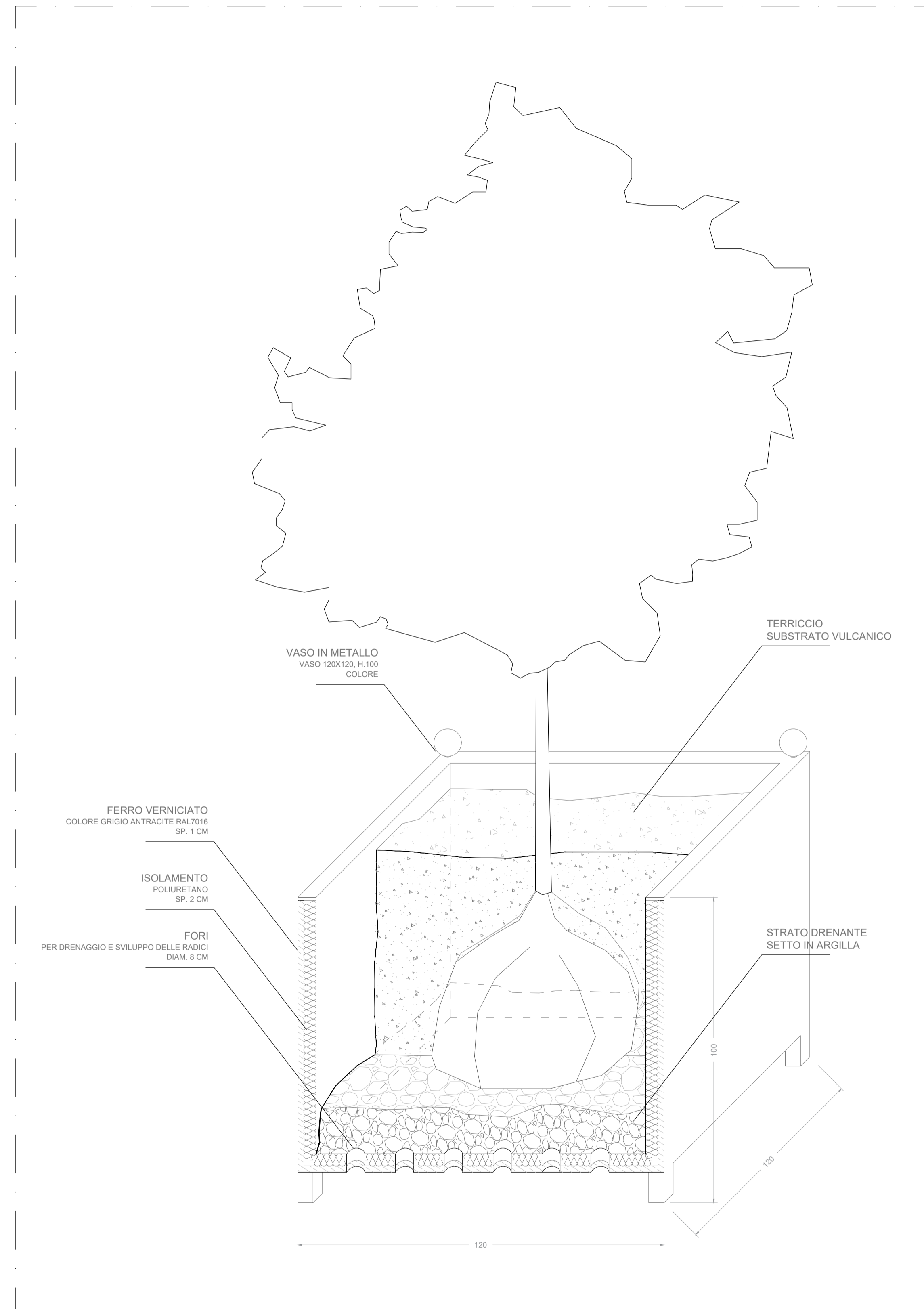
ESPLOSO ASSONOMETRICO - DETTAGLIO FIORIERA 1:10
